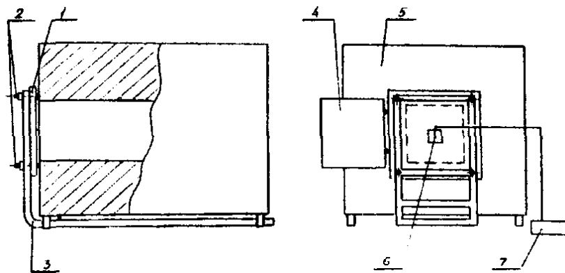
Рис. 5. Принципиальная схема установки для определения устойчивости пакета
