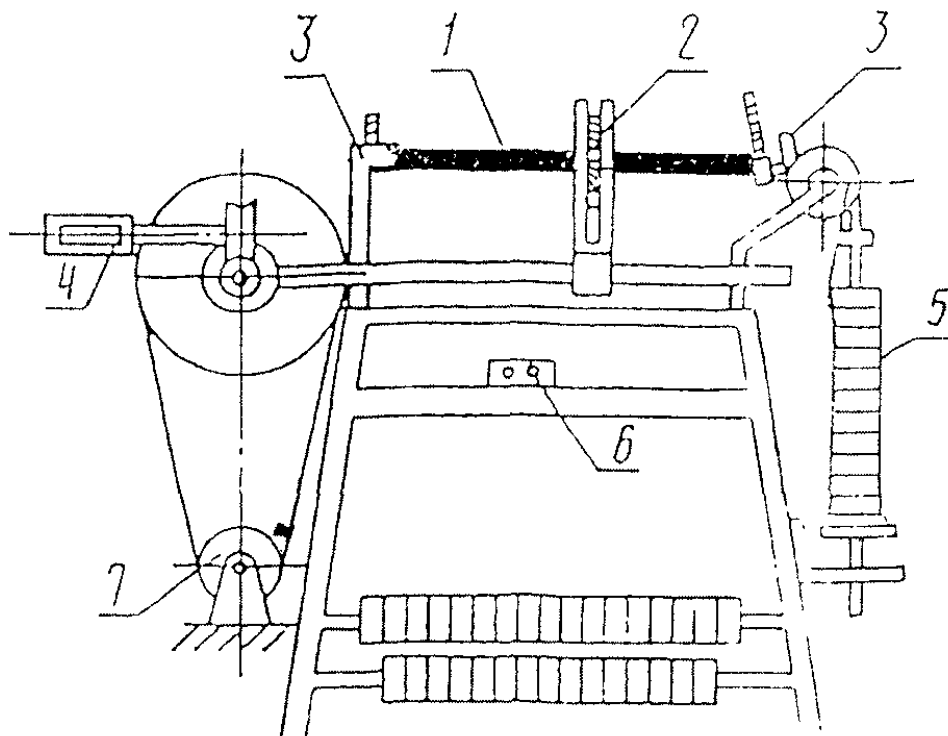
Рисунок 9. Принципиальная схема установки по определению устойчивости материалов к истиранию:
