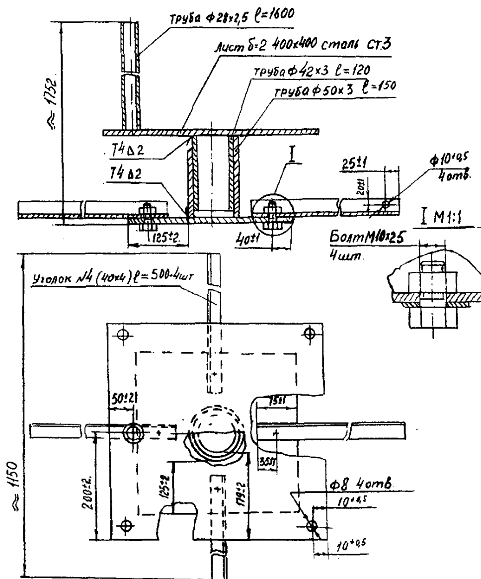
Рис. А. 1. Стенд для термических испытаний
